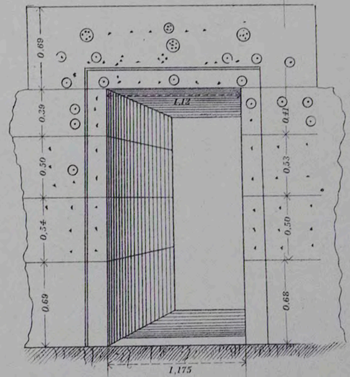
Θύρα τοῦ θαλάμου Κλίμαξ 1:50
